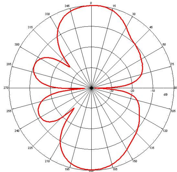
E-PLANE
