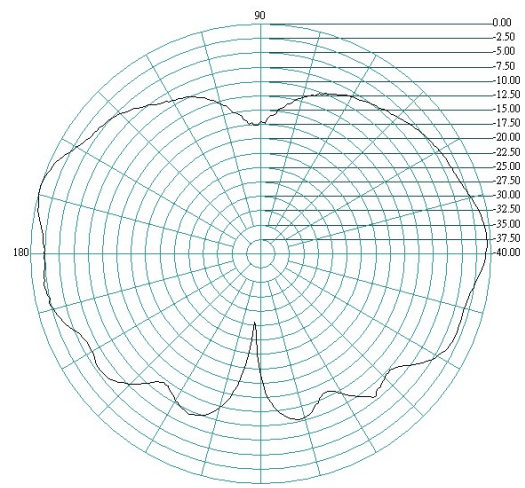
E-PLANE
