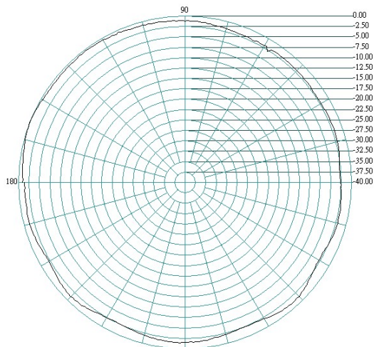
H-PLANE
