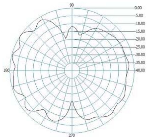
E-PLANE
