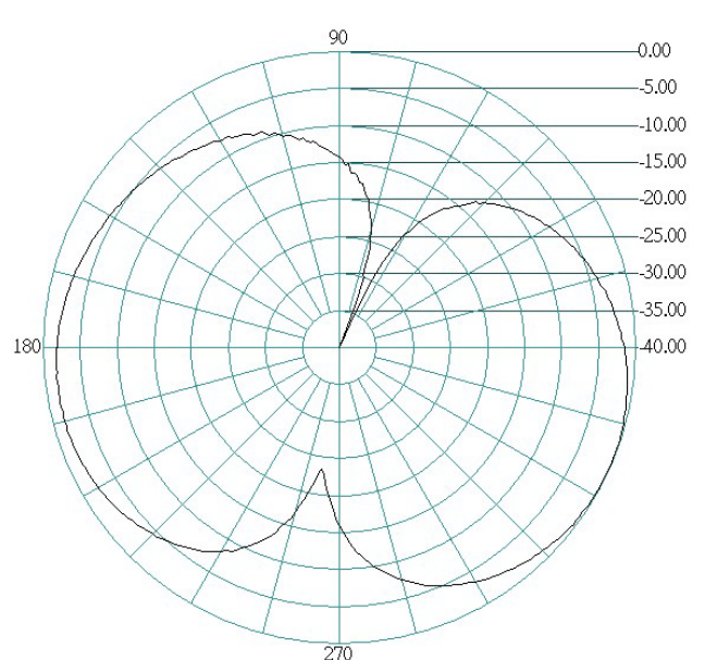
E-PLANE
