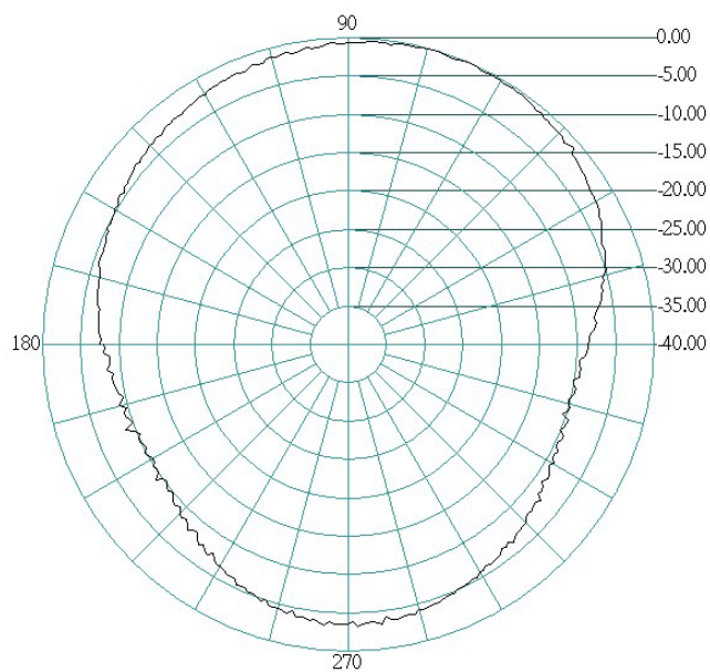
H-PLANE
