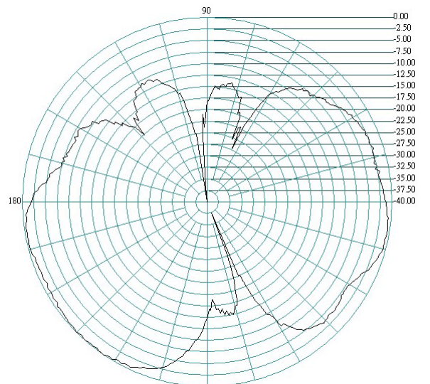
E-PLANE
