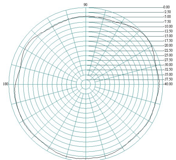
H-PLANE
