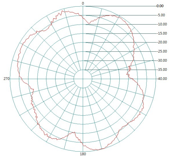
E-PLANE
