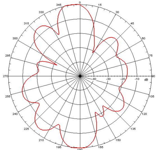
E-PLANE
