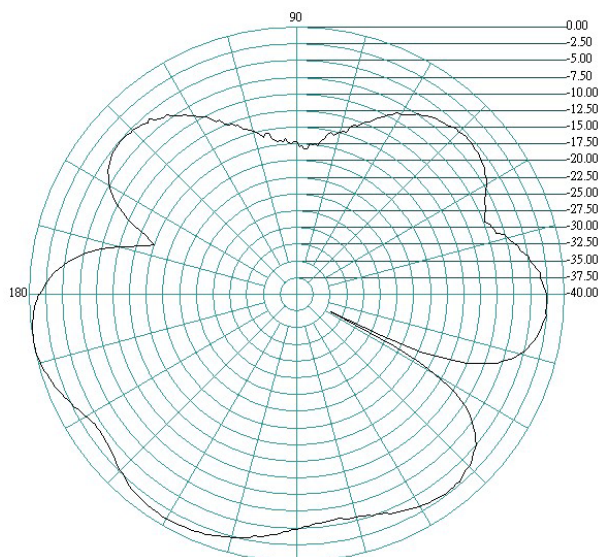
H-PLANE
