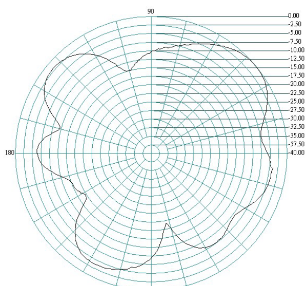
E-PLANE
